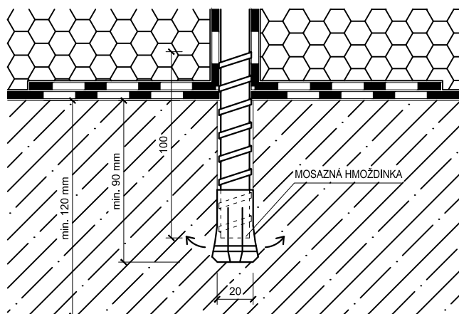
KOTVENÍ POMOCÍ MOSAZNÉ HMOŽDINKY (M1:3)
